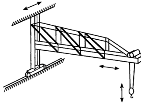
Fig. 5 Wall Crane
